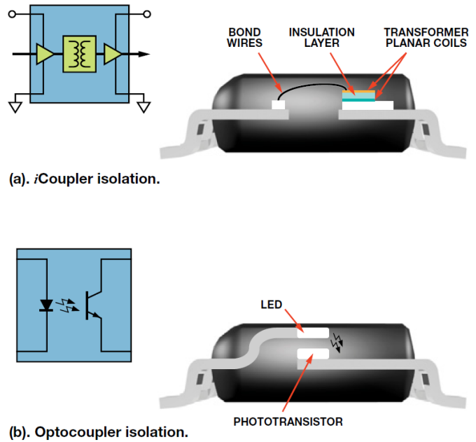
图 4. 隔离技术比较
