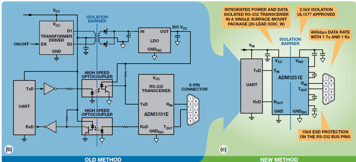
图 8. 单通道 RS232 收发器应用 (a) ADM3251E 规格 (b) 传统方法 (c) iCoupler + isoPower 方法
