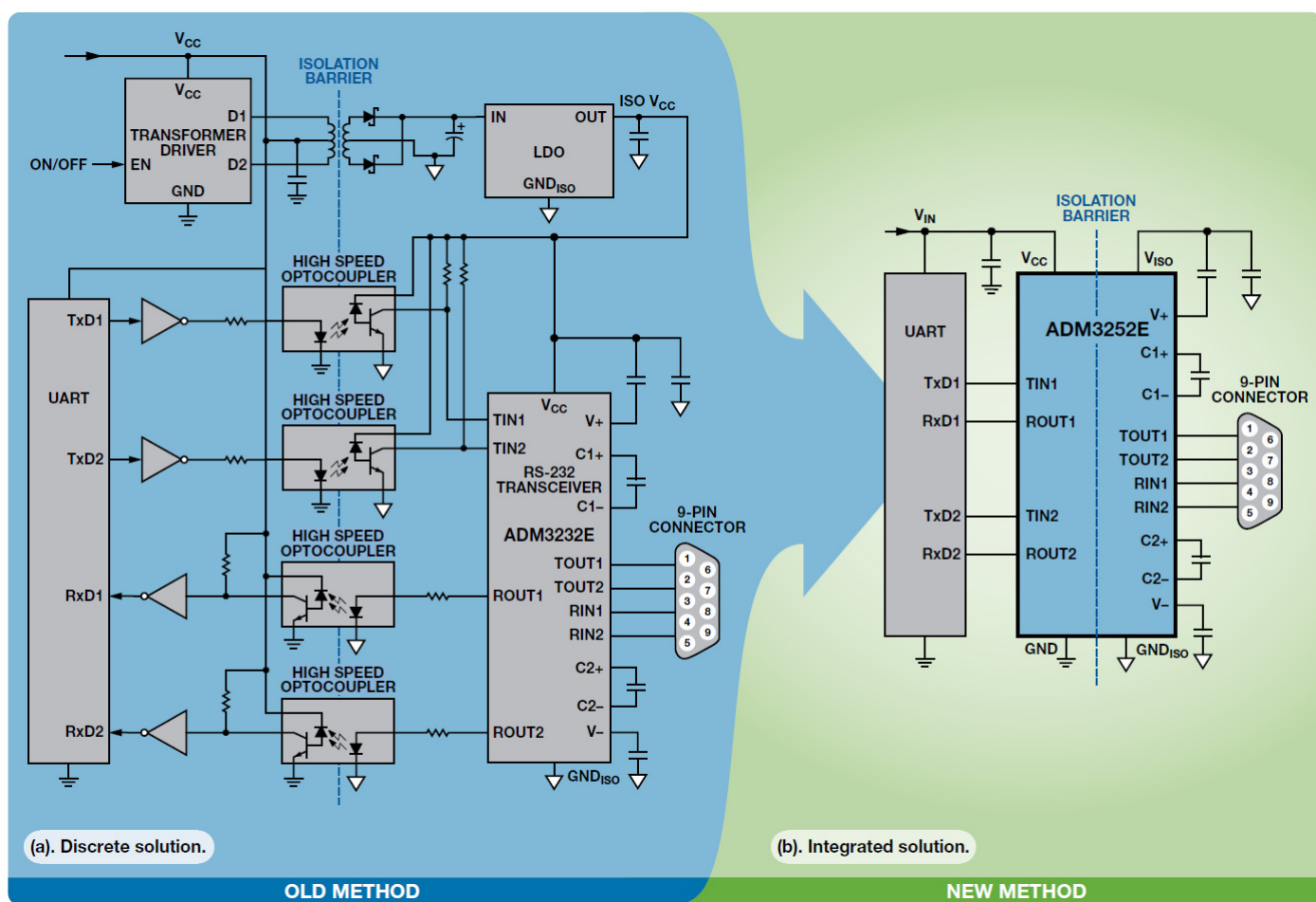
图 5. 隔离式 RS-232 设计比较
